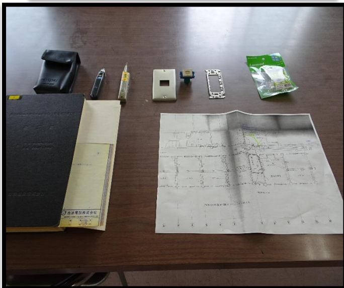
【生徒会室配線図・道具等】
